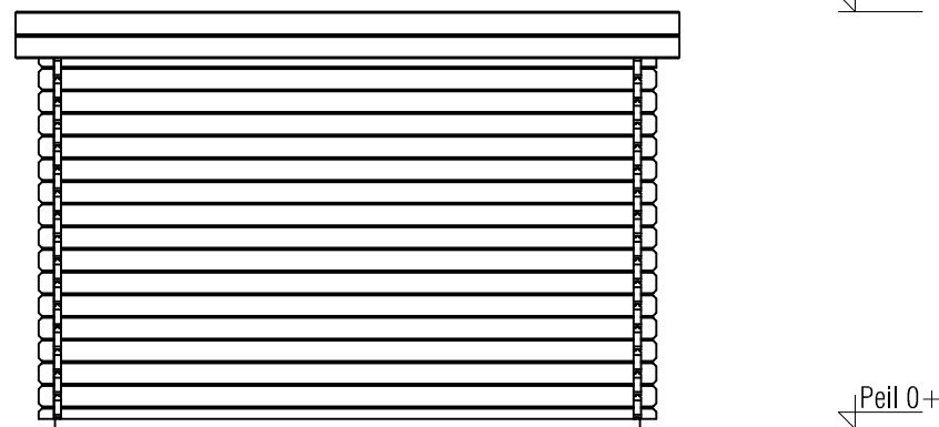
Achteraanzicht / Rear view / Hinterseite
