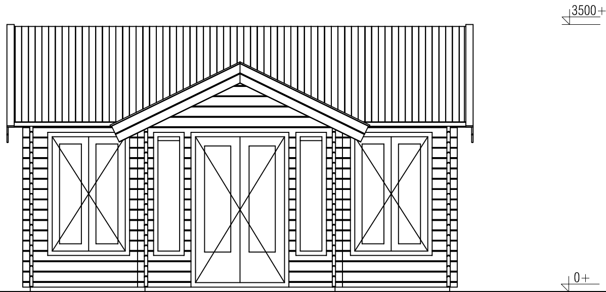
Voorraanzicht / Front view / Vorderansicht
